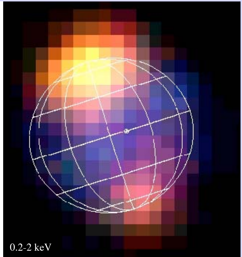
XMM-Newton
